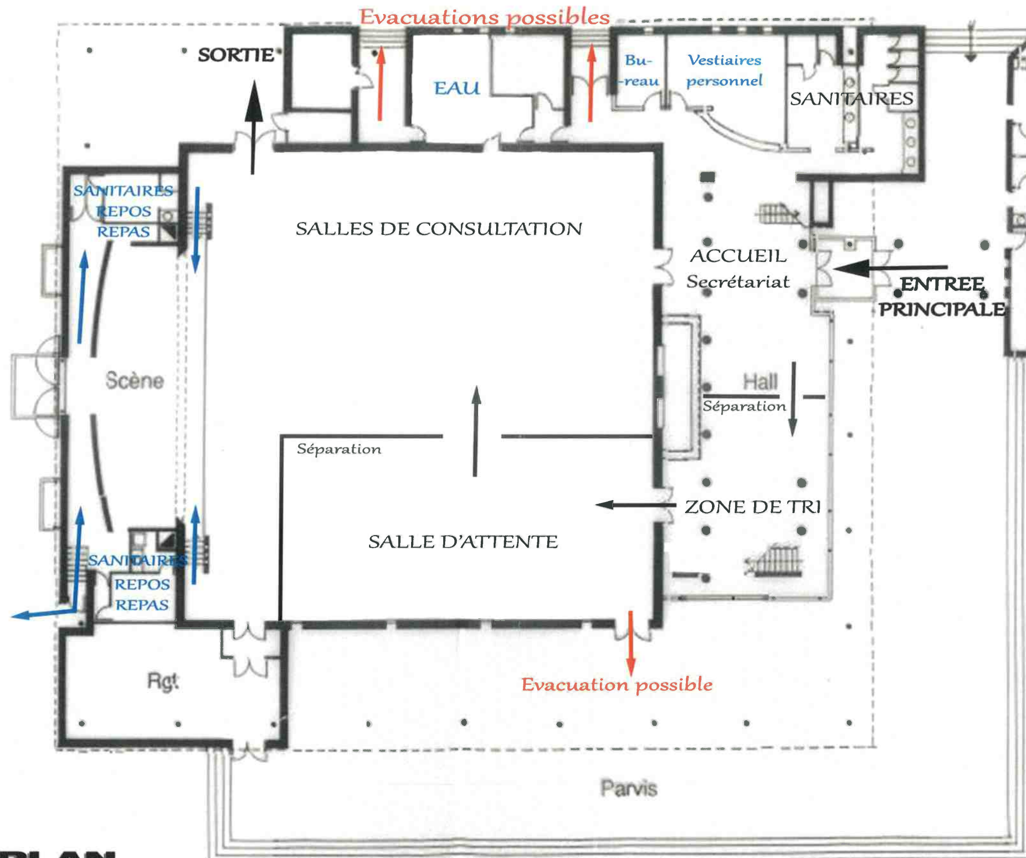
PLAN Salle des Fêtes Rez-de-chaussée
